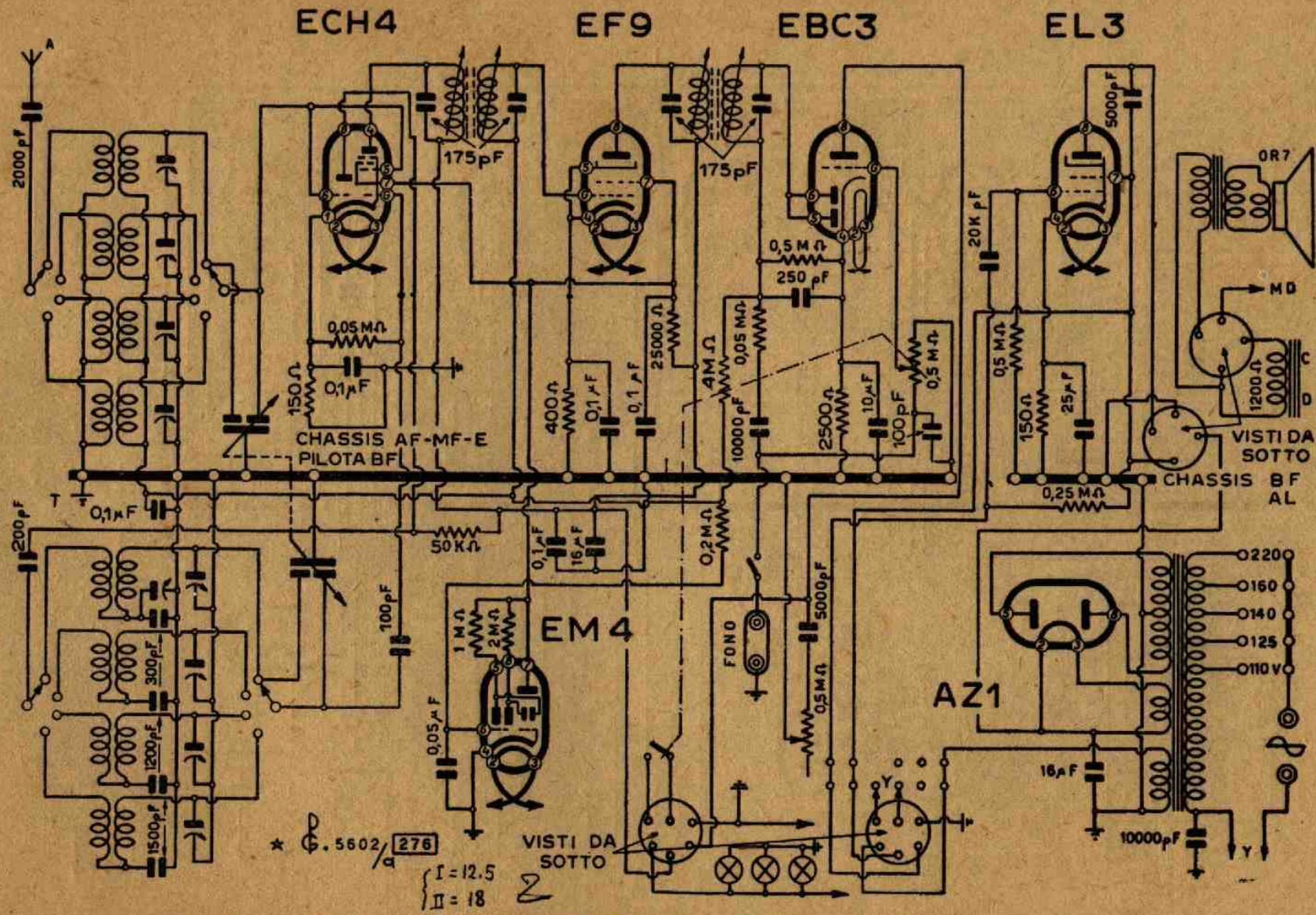
Lo schema elettrico del mod. 642 R della O. R. E. M. (Corso Ticinese, 1 - Milano).
